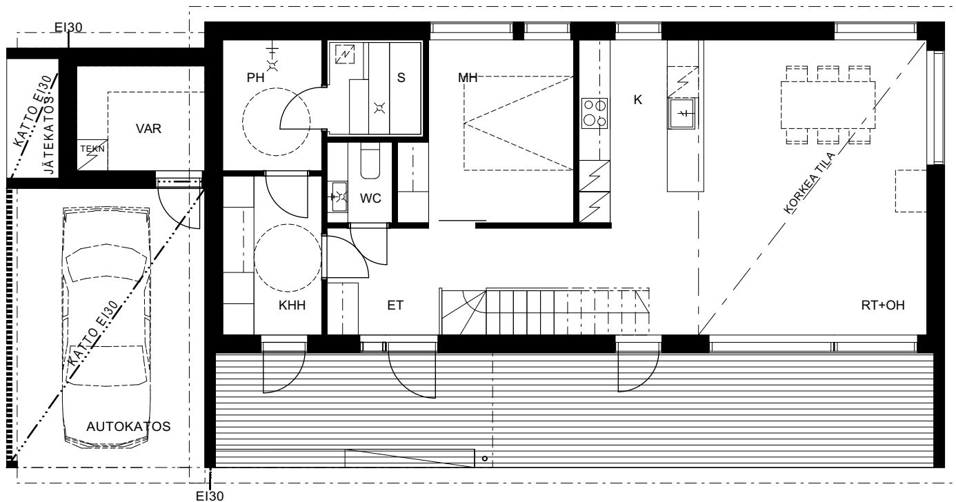
POHJAPIIRROS 1.-KERROS
