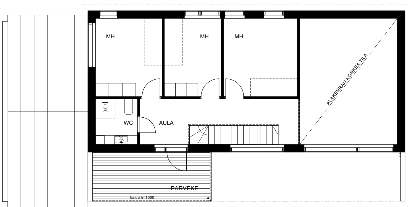
POHJAPIIRROS 2.-KERROS
