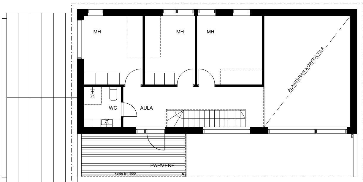
POHJAPIIRROS 2.-KERROS
