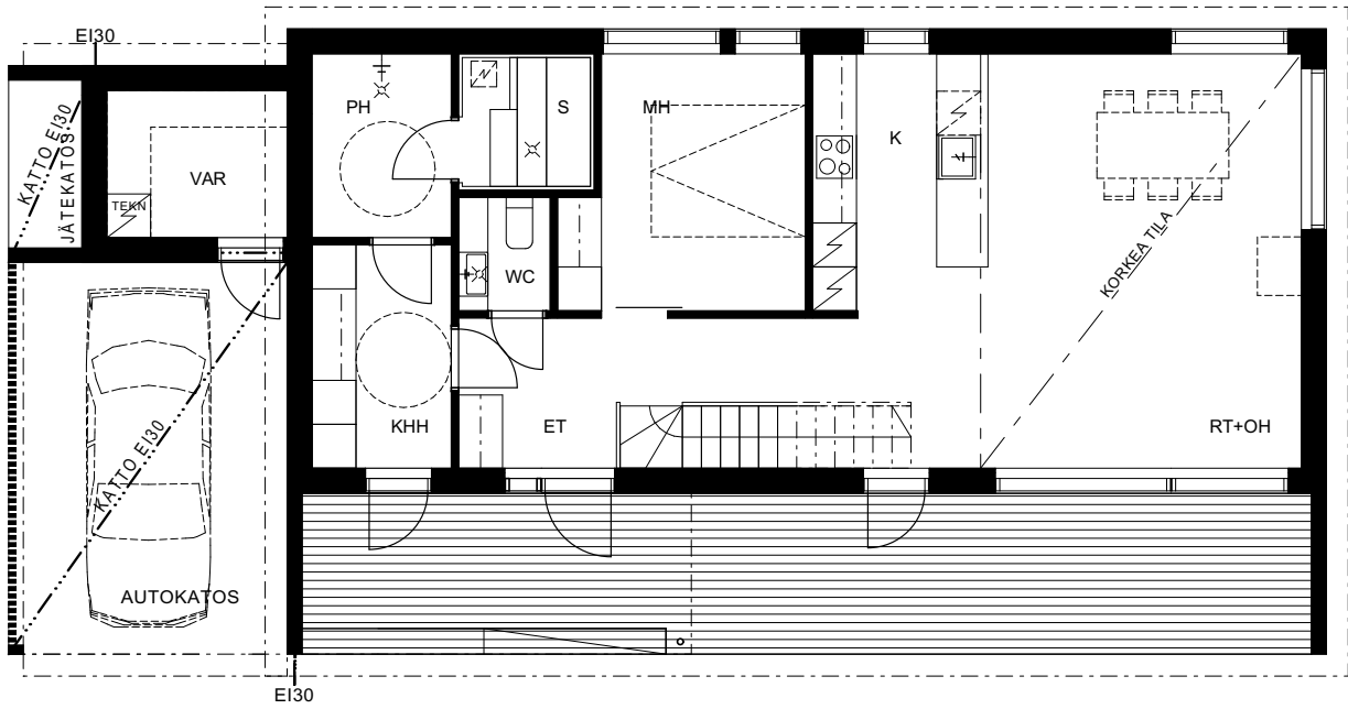
POHJAPIIRROS 1.-KERROS
