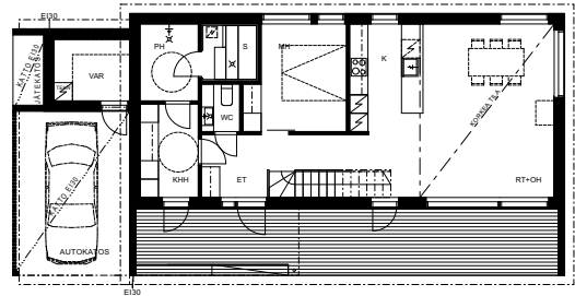
POHJAPIIRROS 1.-KERROS
